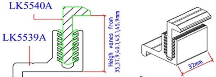
Type 1 FLEXIBLE Z CLAMP LK5539A & LK5540A Length : 32 mm Finishing : M.F
