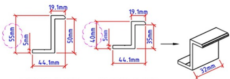
EDGE Z CLAMP LK5279 Scale 1:3 Length : 32 mm Finishing : M.F
