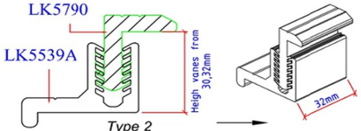
Type 2 FLEXIBLE Z CLAMP LK5539A & LK5790 Length : 32 mm Finishing : M.F
